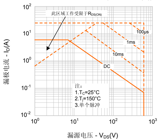
图9-1. 最大安全工作区域(SVF6N60F(G))
